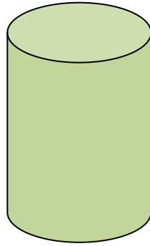
κύλινδρος
