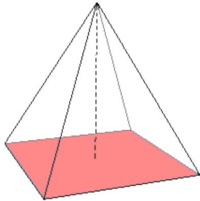
πυραμίδα
