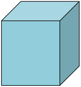
κύβος
